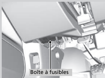
Modèle à conduite à droite
