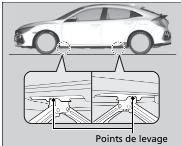
Points de levage
